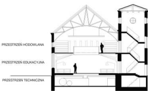
PRZEDKÓJ SKALA 1:200
