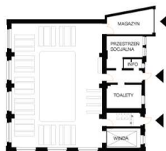
RIZUT PASTERU SKALA 1:200
