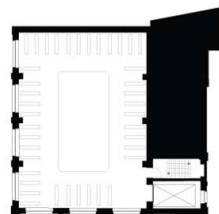
RIZUT PIĘTROWEGO PIĘTRA SKALA 1:200
